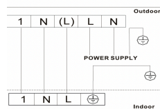
Електрическа схема
